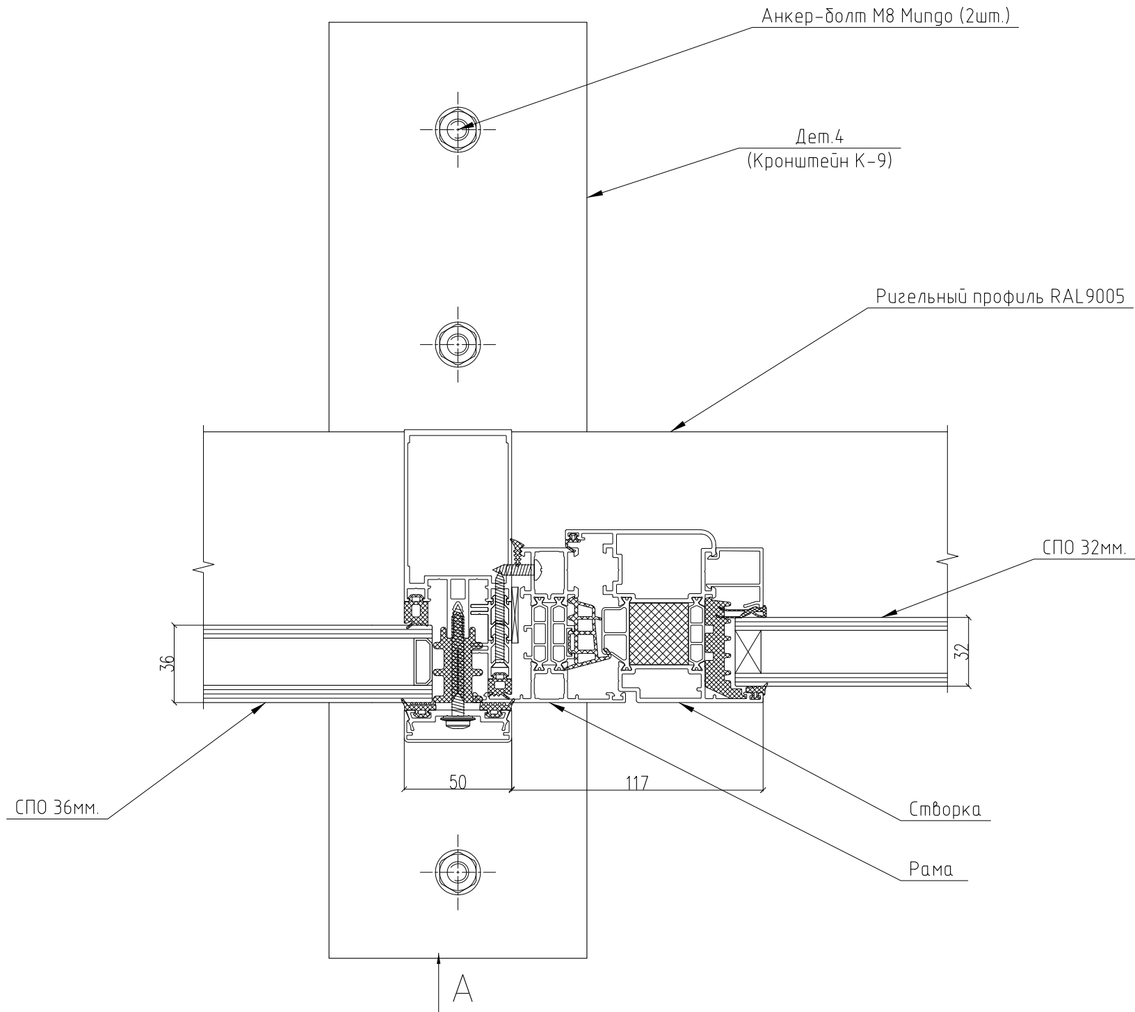
Вид А
