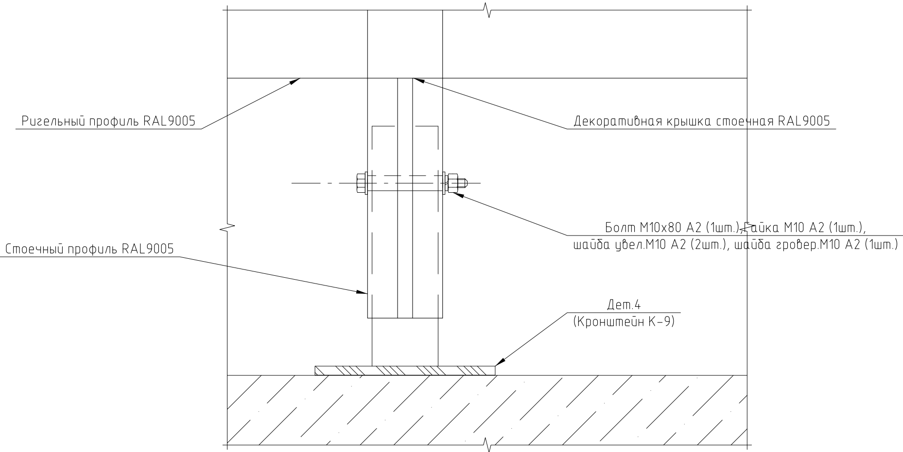
Вид А
